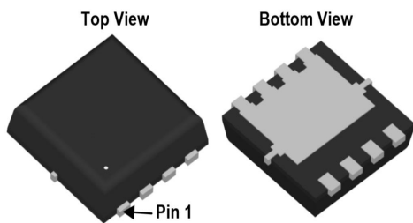
PDFN5X6-8L
